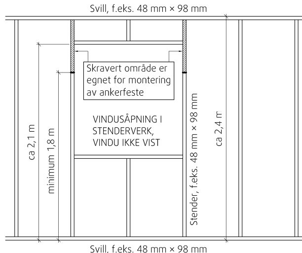
Fig. 7 Oppriss av typisk stendervegg, anbefalte områder for feste av forankring til parat redningsline
