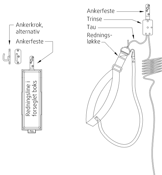
Fig.1 Forseglet boks
