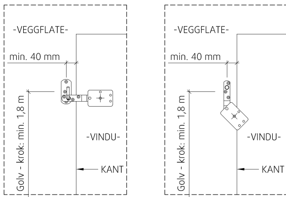
Fig. 5. Med ankerkrok.
